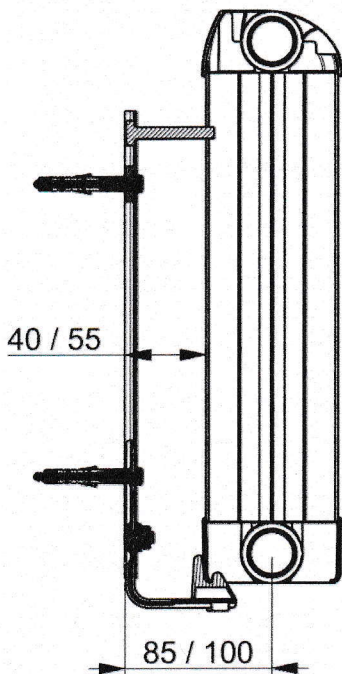
Prerez A-A
